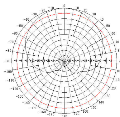
H-Plane
