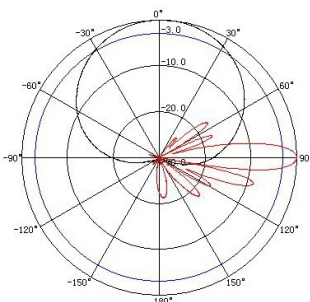
870~960MHz: ±45° Pol.
