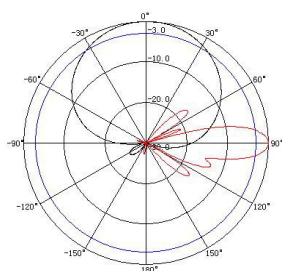
870~960MHz: ±45° Pol.
