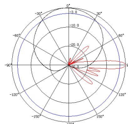
1850~1990MHz: ±45° Pol.
