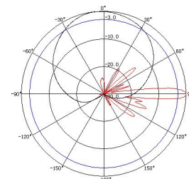
1920~2170MHz: ±45° Pol.
