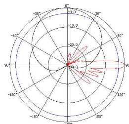
1710~1880MHz: ±45° Pol.
