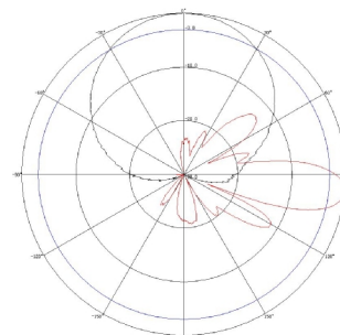
1920~2170MHz: ±45° Pol.
